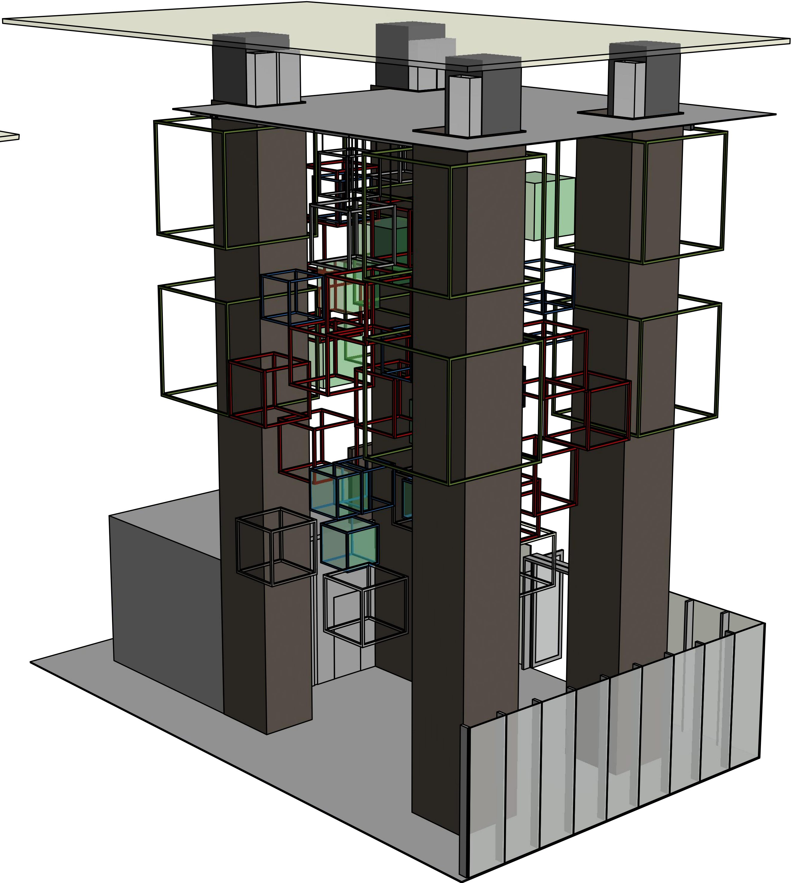
ISOMETRIC BACK 15 SCALE: 1/50
